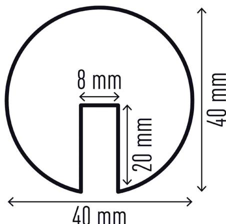
Detailansicht: Maße Kantenschutzprofil E8R
