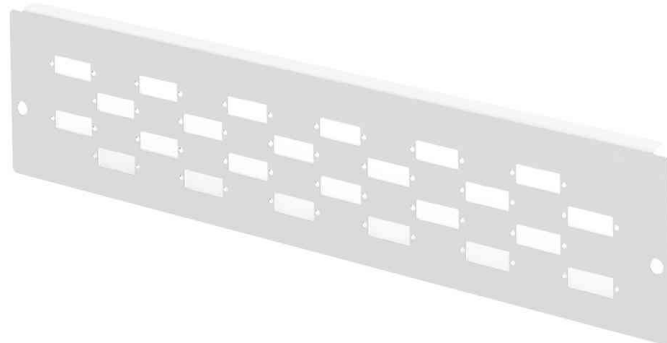
Adapterplatte für Unibox Medium (DN-96802M-2)
