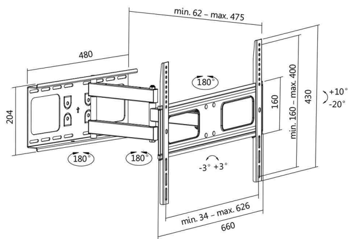
TV-Wandhalterung 11115860 - Abmessungen
