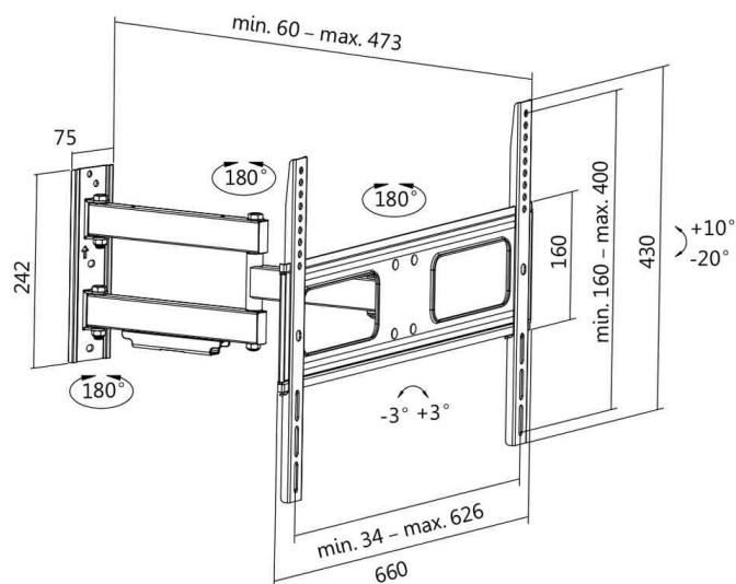
TV-Wandhalterung 11115851 - Abmessungen
