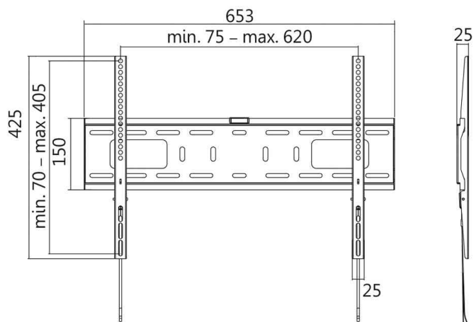
TV-Wandhalterung - Abmessungen
