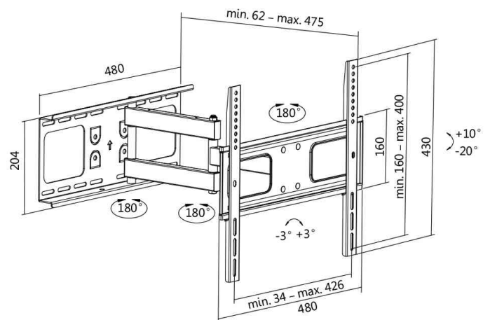
TV-Wandhalterung 11115847 - Abmessungen
