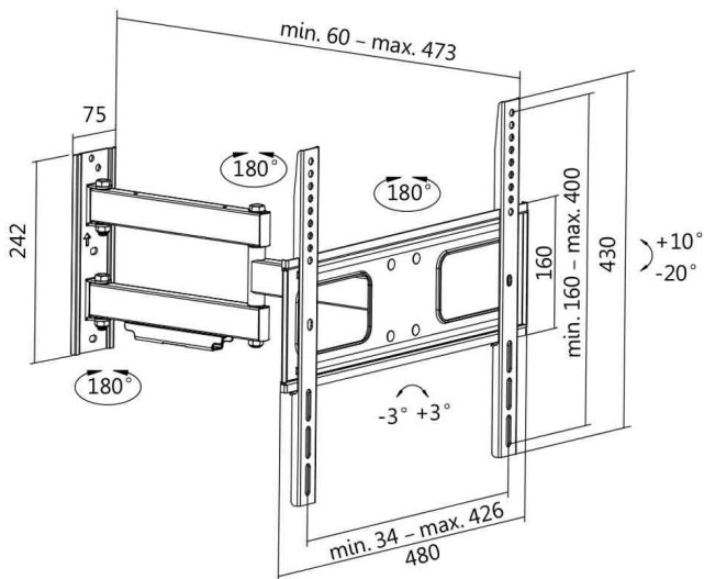
TV-Wandhalterung 11115846 - Abmessungen
